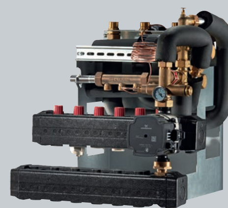
DRe-Skakt Fuldisolieret fordelermodule til fordelere for gulvarmekreds, til anvendelse i installationskake
