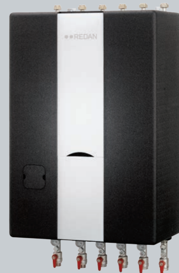
Akva Lux II VXi med isoleringsfront Fuldisoleret unit for varme og varmt vand, til indirekte anlæg. Rør op og ned
