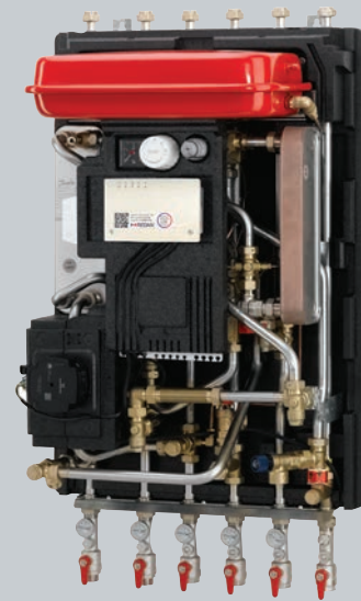
Akva Lux II VXi Fuldisoleret unit for varme og varmt vand, til indirekte anlæg. Rør op og ned
