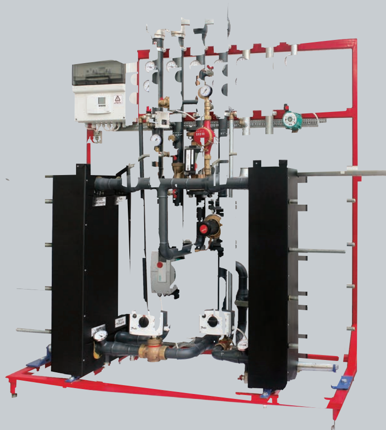
Red Frame Gulvstillet unit til varme og varmt vand - med svejste rør og boftede pladevarmevekslere
