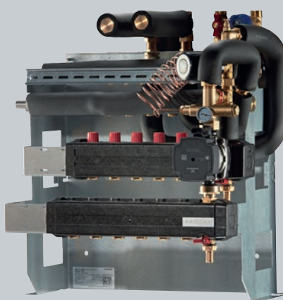
DRe-GI Fuldisolieret fordelermodule til fordelere for gulvarmekreds inklusiv shunt med pumpe og termostat for gulvarme
