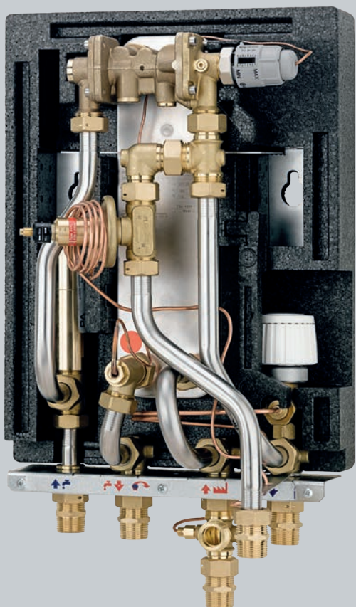
Akva Lux II TDv Fuldisolert unit for varme og varmt vand til direkte anlæg, med AVE trykdiligner
