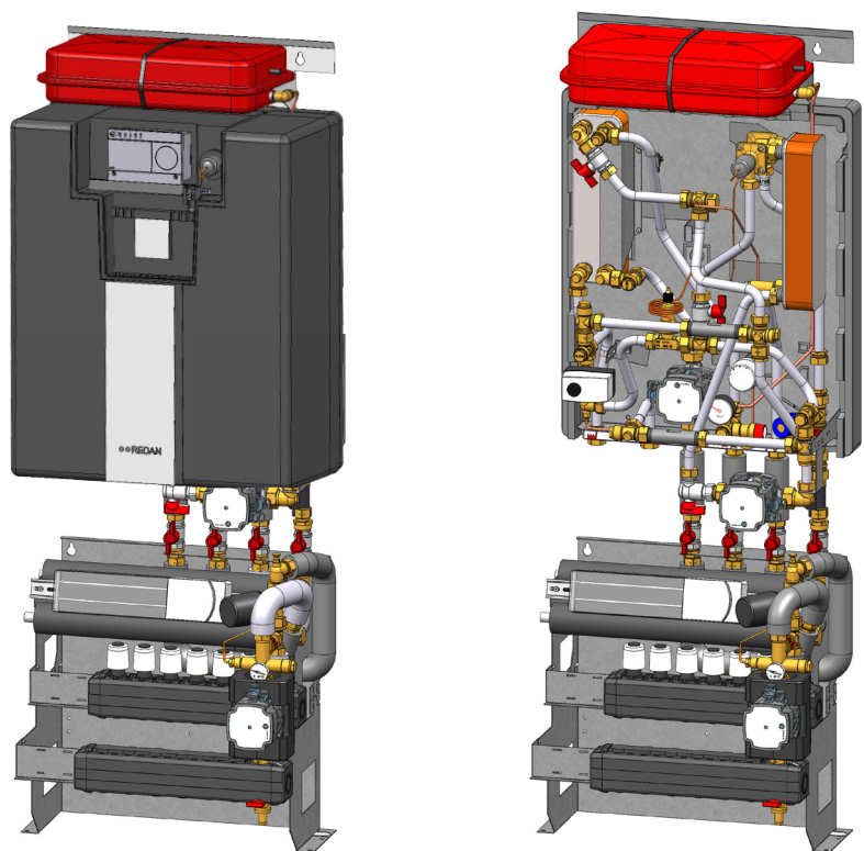
Akva Lux II VXe med boostersæt og DRe fordelemodule
