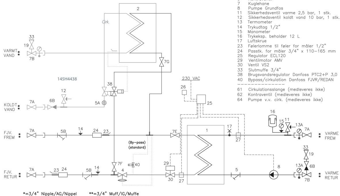
MODEL: Akva Lux VXe Solo
